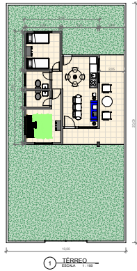
1 TÉRREO ESCALA: 1:100
