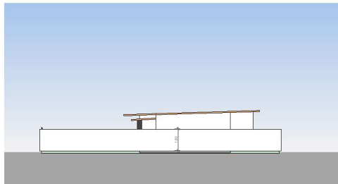
6 FACHADA LESTE ESCALA: 1:100
