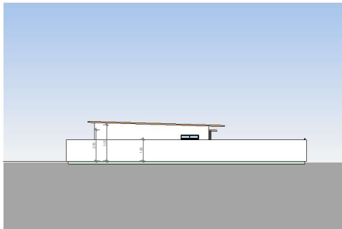
4 CORTE A ESCALA: 1:100
