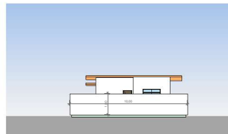
7 FACHADA NORTE ESCALA: 1:100
