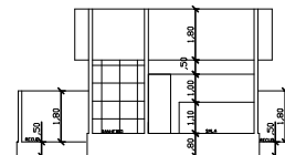
CDRTE TRANSVERSAL BB ESCALA 1 / 100
