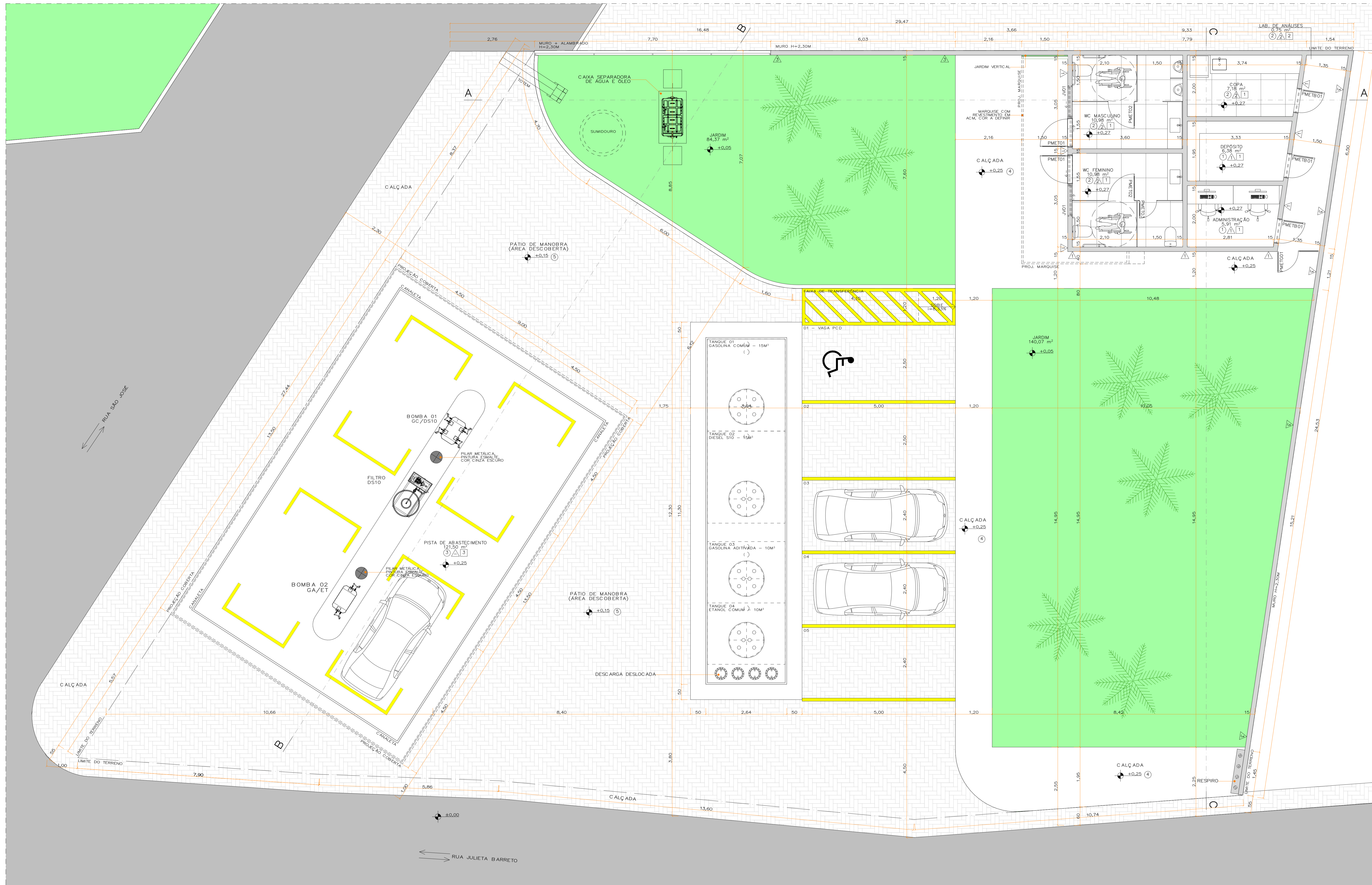
PLANTA BAIXA - TERREJO POSTO DE COMBUSTÍVEL 1:50
