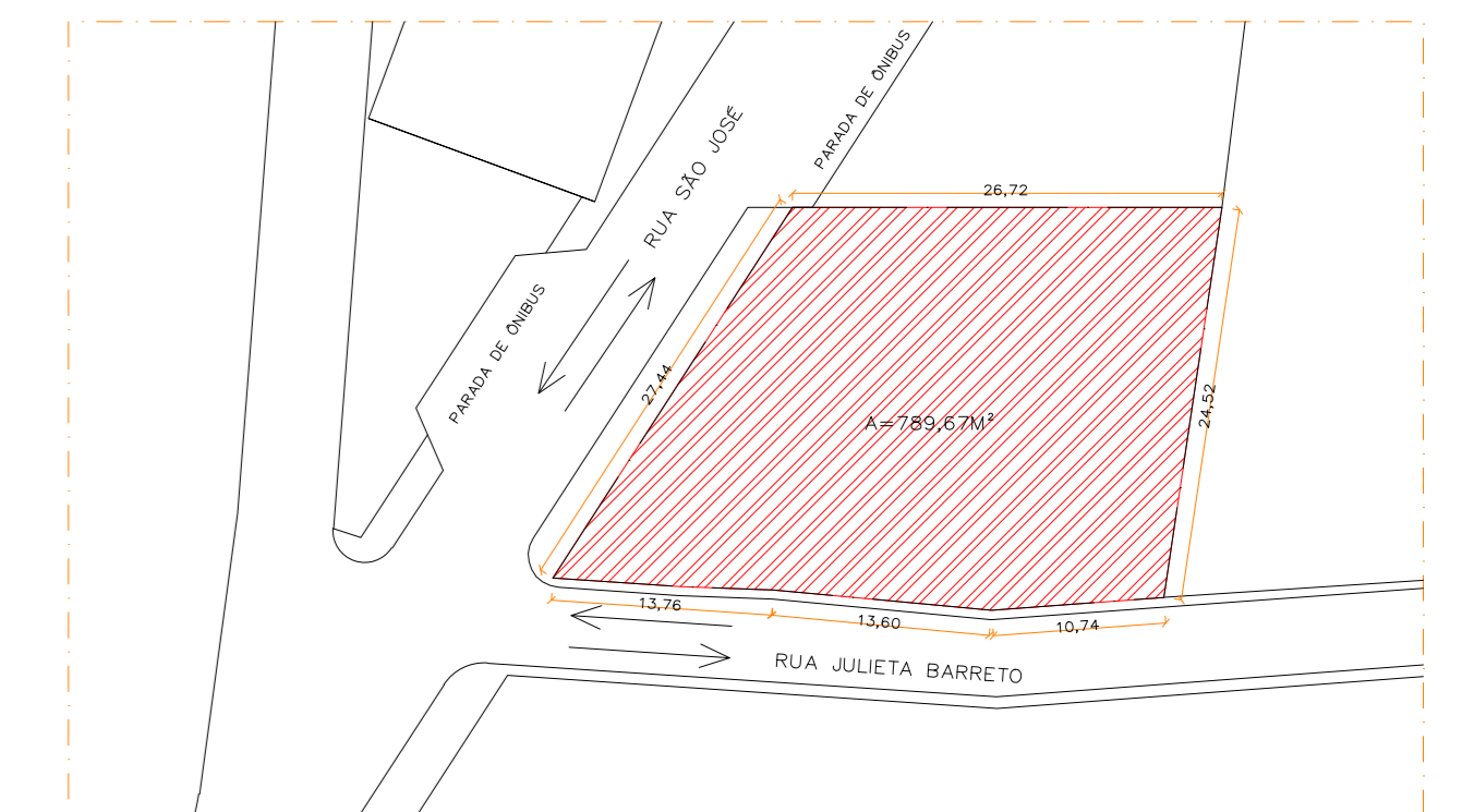
PLANTA DE SITUAÇÃO POSTO DE COMBUSTÍVEL
