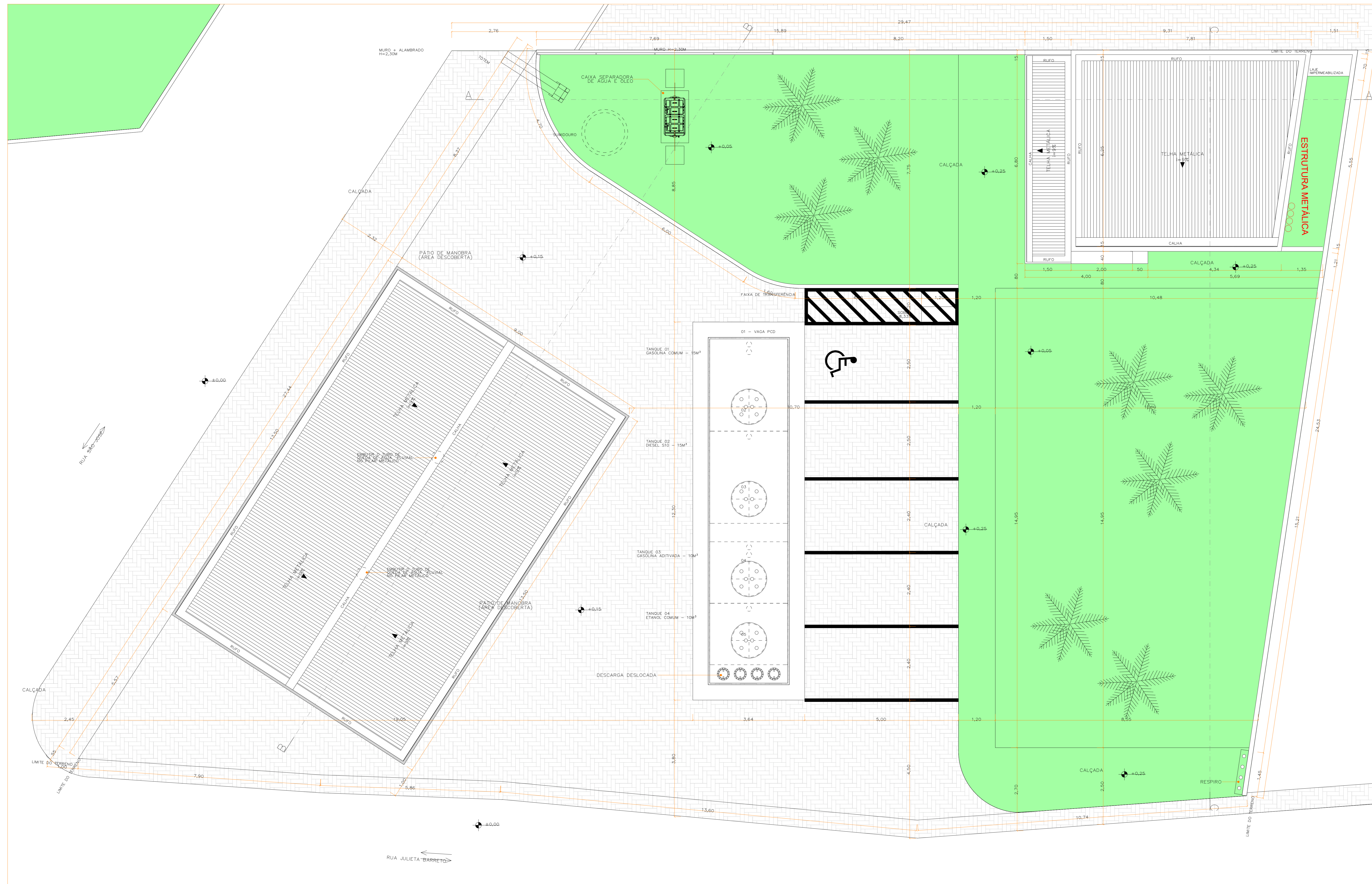
PLANTA DE COBERTA E LOCAÇÃO POSTO DE COMBUSTÍVEL 1:50
